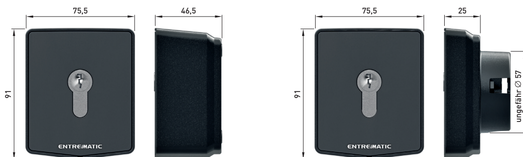
AXK5M - AXK5NM (prevedenie bez cylindrickej vložky)
